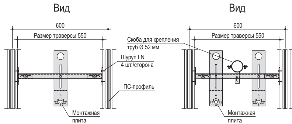
Горизонтальная проекция
